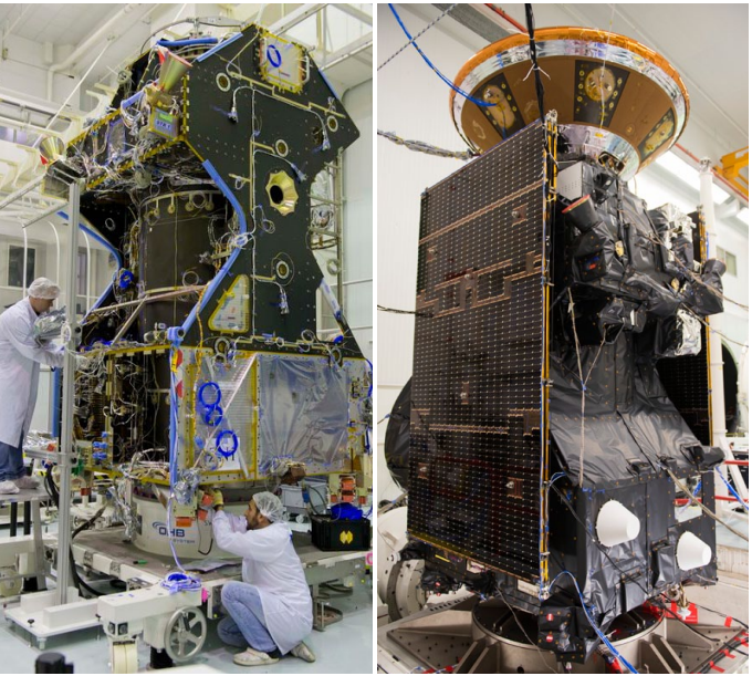
Spurengas-Orbiter: Design, Fertigung und Test. Fotos: ESA (S. Corvaja bzw. A. Le Floch)/ Trace Gas Orbiter: design, manufacturing and test. Photos courtesy ESA (A. Le Floch & S. Corvaja)
