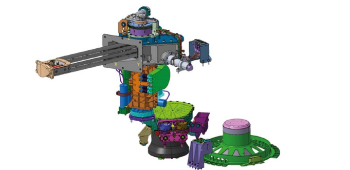
Das Probenaufbereitungs- und -verteilsystem (SPDS) für den ExoMars Rover setzt sich aus vier Mechanismen von OHB zusammen / The Sample Preparation and Distribution System (SPDS) for the ExoMars Rover is made up of four mechanisms by OHB
